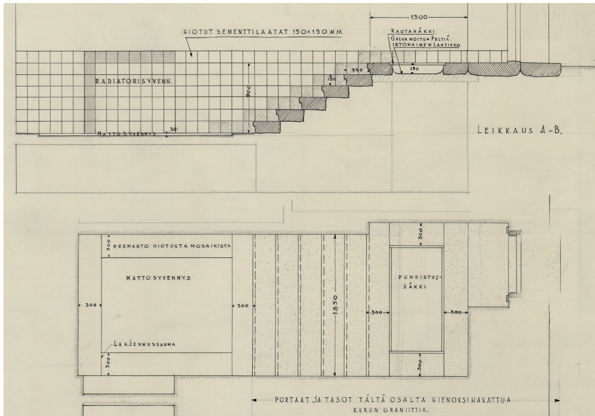
Keskuskäymälän pohjapiirustus ja leikkaus sisäänkäynnin kohdalta. Tampereen kaupungin rakennustoimisto arkkitehtiosasto 1931. TKA
