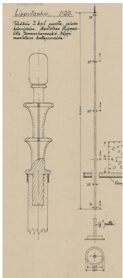
Lipputangon piirustus. Vilho Kolho 1951. TKA
