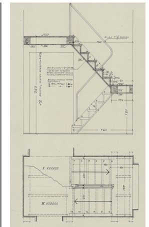
Maistraatin arkisto kaupungintalossa, porraspiirustus. 25.11.1943 TKA
