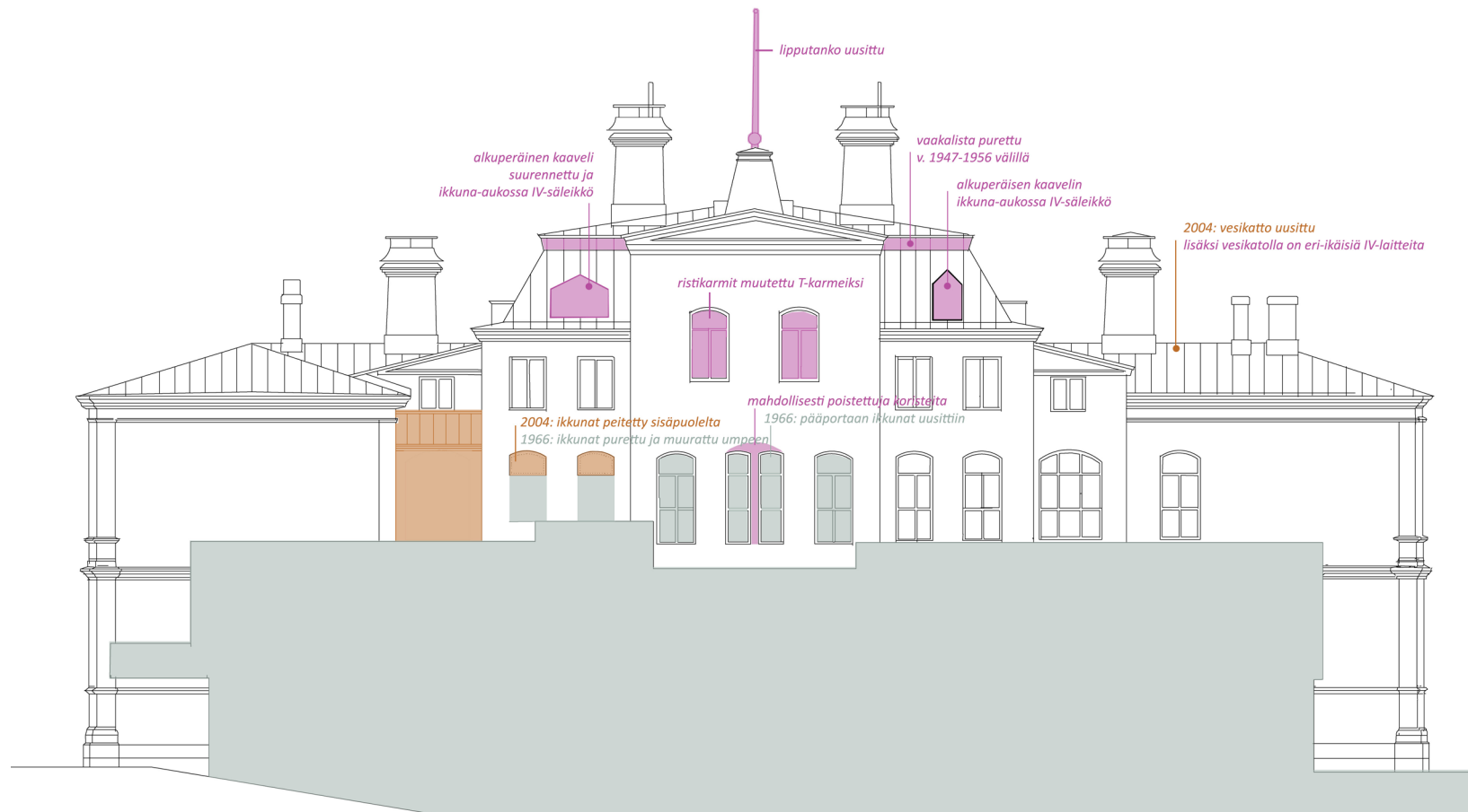
Länsijulkisivun säilyneisyyskaavio
