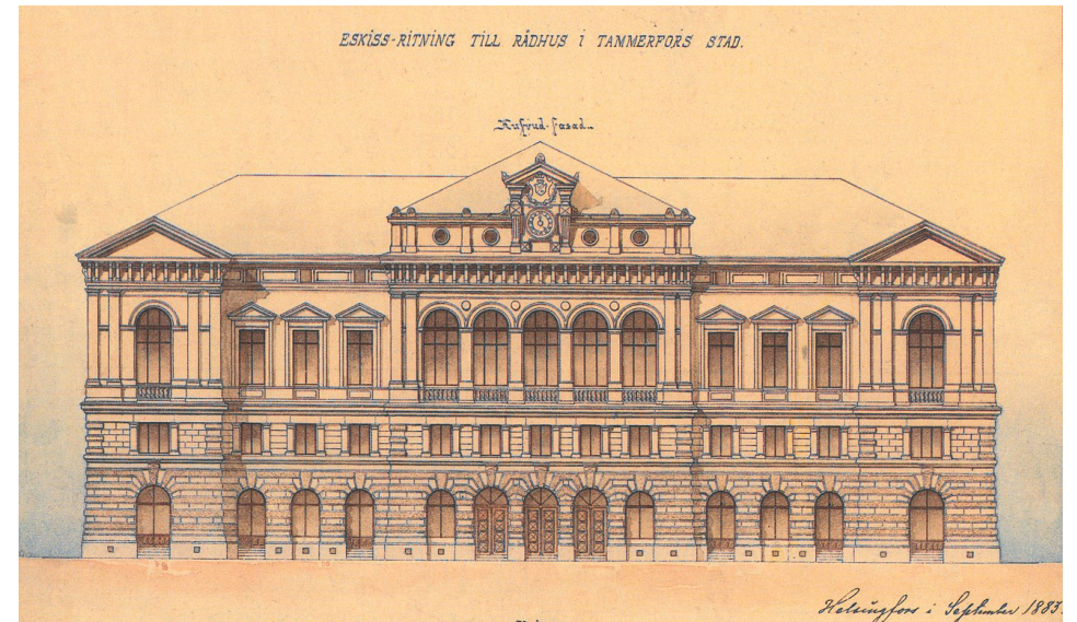
Yllä: Theodor Deckerin toteutumaton suunnitelma raatihuoneesta vuodelta 1885. Suunnitelma edustaa hankkeesta esitettyjä kolmikerroksisia ratkaisumalleja, joissa hallintotoiminnot on sijoitettu ylimpään kerrokseen ja katutasossa on liikehuoneistoja. Välikerros on matala ja osoitettu varastotiloiksi. Kuva kirjasta Järvelä 2007, s. 24.
