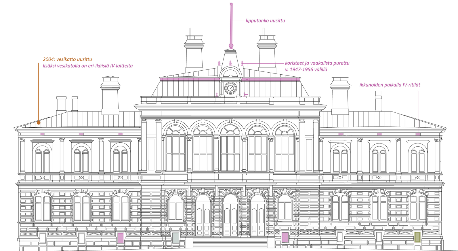
Itäjulkisivun säilyneisyyskaavio
