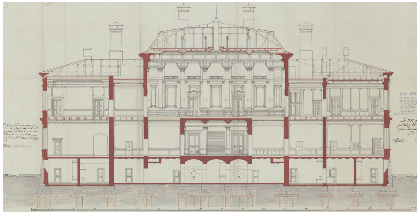
→ → Leikkaus C-D. 1887. RAVA
