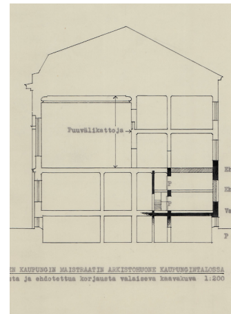
Tampereen kaupungin maistraatin arkistohuone kaupungintalossa ensimmäisessä kerroksessa, muutosehdotus. Pohjapiirros sekä rakennuksen poikkileikkaus, johon merkitty uudet kattorakenteet ja palo-ovet. 15.10. 1942. TKA
