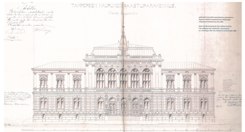
Alla: Georg Schreckin toteutunut suunnitelma raatihuoneesta vuodelta 1886. Suunnitelman keskeisenä erona ja menestystekijänä oli rakennuksen 2-kerroksisuus ja siten pienemmät rakennuskustannukset sekä erityisesti molempien kerrosten tilojen osoittaminen kokonaan hallintotiloiksi. Kuva kirjasta Järvelä 2007, ss. 26-27.
