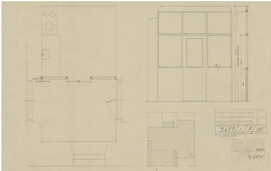
Kaupungintalo. Vankilanhoitajan asunnon keittiön lasiseinä. Keittiön pohjapiirros ja lasiseinä edestä. suunnitellut Vilho Kolho, piirtänyt H. S:mi 1951. TKA
