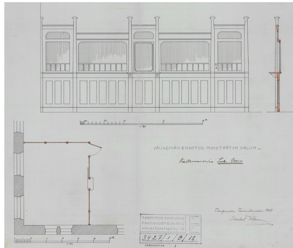
Väliseinäehdotus maistraatin saliin (eli tähän aikaan 2. kerroksen eteläiseen saliin). Lambert Petterson 1904. TKA
