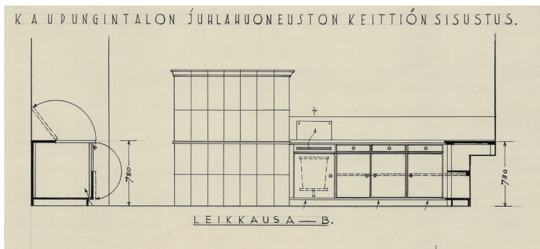
Kaupungintalon juhlahuoneiston keittiön sisustus. E. A. L. 20.7.1931 TKA
