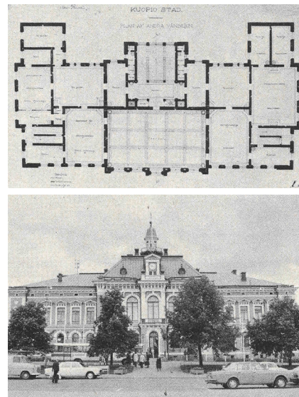
Kuopion kaupungintalo. Pohjapiirustus pääkerroksesta, valokuvat pääjulkisivusta ja juhlasalista. Kuvat kirjasta Lilius 1983, s. 184-185
