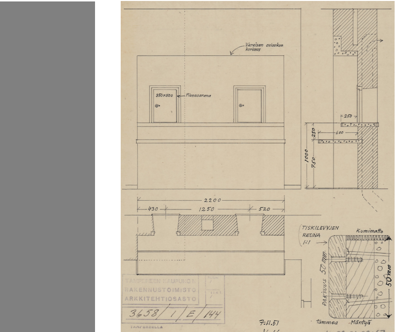
Liikennelaitoksen toimipaikka kaupungintalossa. Lippukassaluukut. Vilho Kolho 1951 TKA
