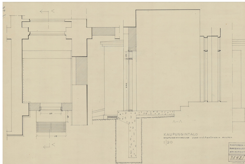
Kaupungintalo, kaupunginvankilan ulko-sisäänkäynnin muutos. Kaupunginvankilan uloskäynnin pohjapiirustus, leikkaus A-A ja ulko-oven piirustus. A. S. 1948. TKA
