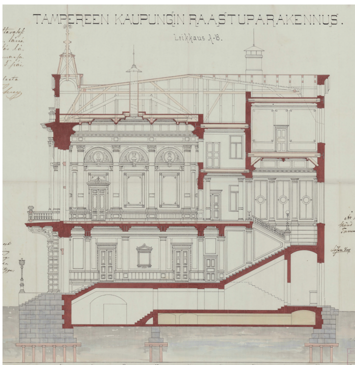
→ → Leikkaus A-B. Georg Schreck syyskuu 1887. RAVA
