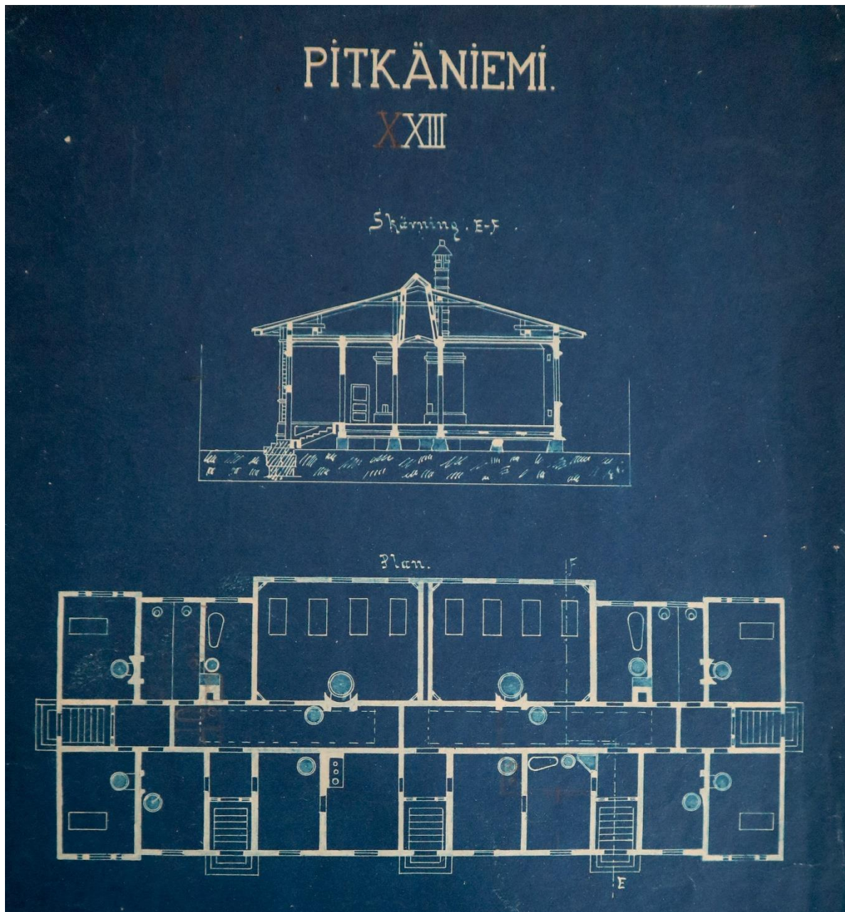
Kuva 32. Rakennuksen 23 alkuperäiset piirustukset. (Lähde: Pirkanmaan sairaanhoitopiirin arkisto.)
