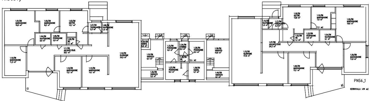
Kuva 26. Rakennuksen 56 eli Toivolan nykyhetkeä kuvaava pohjapiirustus. Rakennus on miltei identtinen rakennus 55:n kanssa, mutta länsipuolen asunnossa on muutamia eroavaisuuksia huonejaossa sekä autotallin jäsentelyssä. (Lähde: Pirkanmaan sairaanhoitopiirin arkisto.)
