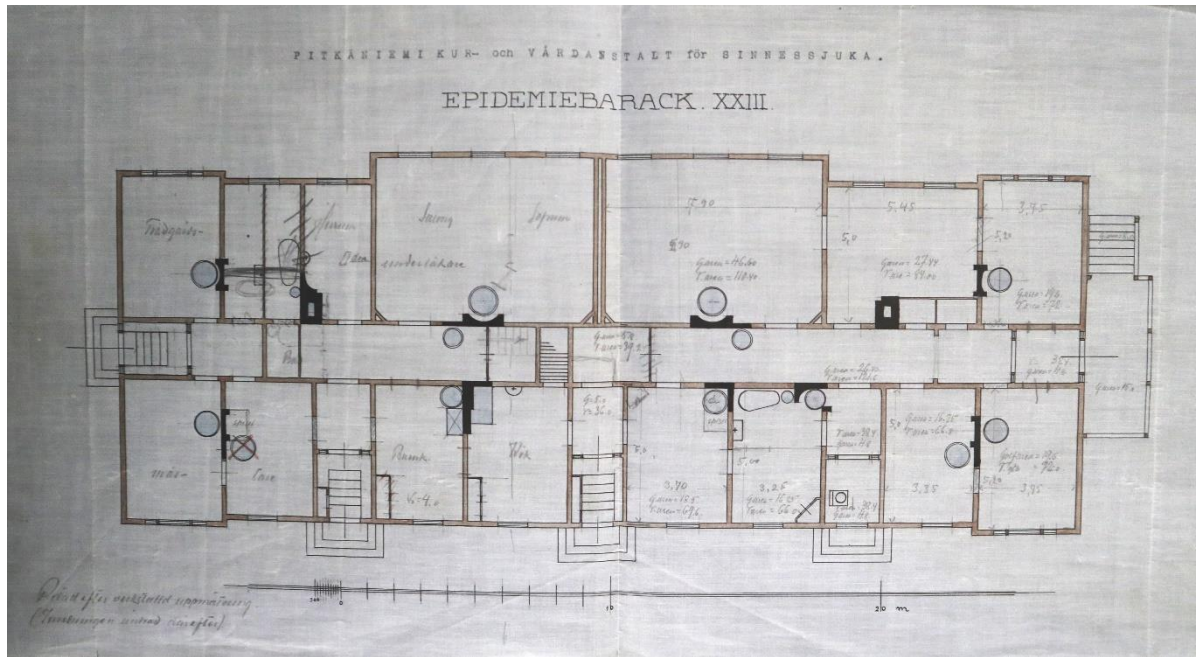
Kuva 33. Epidemiaosaston piirustus. (Lähde: Pirkanmaan sairaanhoitopiirin arkisto.)
