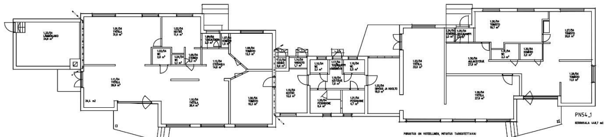
Kuva 24. Rakennuksen 54 nykyhetkeä kuvaava pohjapiirustus. Rakennuksessa sijaitsee työtiloja ja länsipäädyssä lämmönjakuhuone. Kahden asunnon väliin jäänyt autotalli on muutettu pesuhuonetiloiksi, joiden keskeltä kulkeva käytävä yhdistää osat toisiinsa. (Lähde: Pirkanmaan sairaanhoitopiirin arkisto.)
