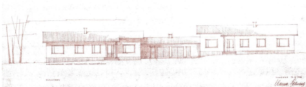
Kuva 21. Piirustus rakennuksen 55 tai 56 pohjoisjulkisivusta vuodelta 1956. (Lähde: Pirkanmaan sairaanhoitopiirin arkisto.)
