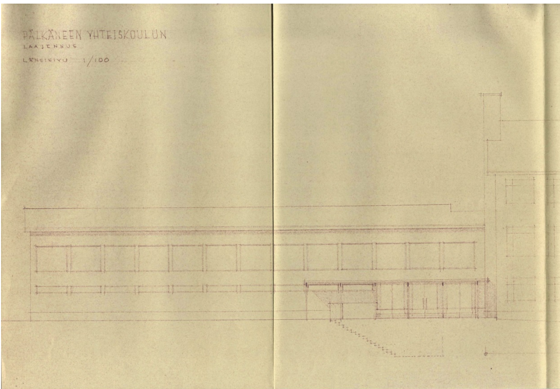
Lupapiirustus vuodelta 1962. Juhlasaliiven laajennus. Julkisivu länteen.
