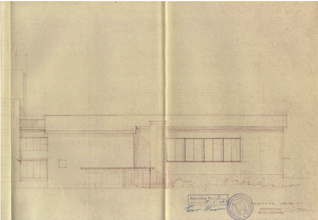
Lupapiirustus vuodelta 1962. Juhlasaliiven laajennus. Julkisivu itään.
