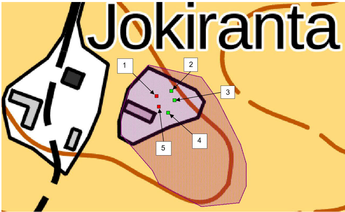
Koekuoppien 1-5 sijainti. Koekuopat 1 ja 5, joista tehtiin havaintoja, on merkitty karttaan punaisella. Pohjakartta (c) Maanmittauslaitos 01/2022. Kirsi Luoto 4.1.2022
