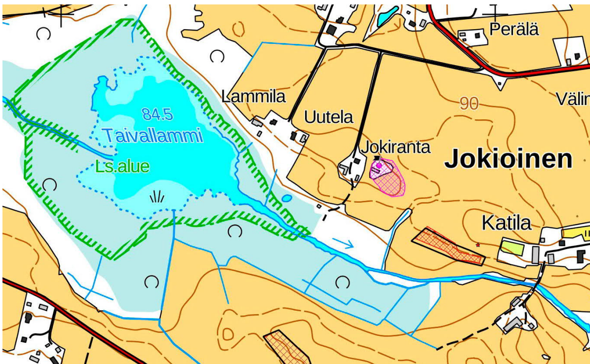
Jokirannan mahdollinen muinaisjäännös on merkitty karttaan aniliinilla aluerajauksella. Pohjakartta (c) Maanmittauslaitos 01/2022 Kirsi Luoto 4.1.2022
