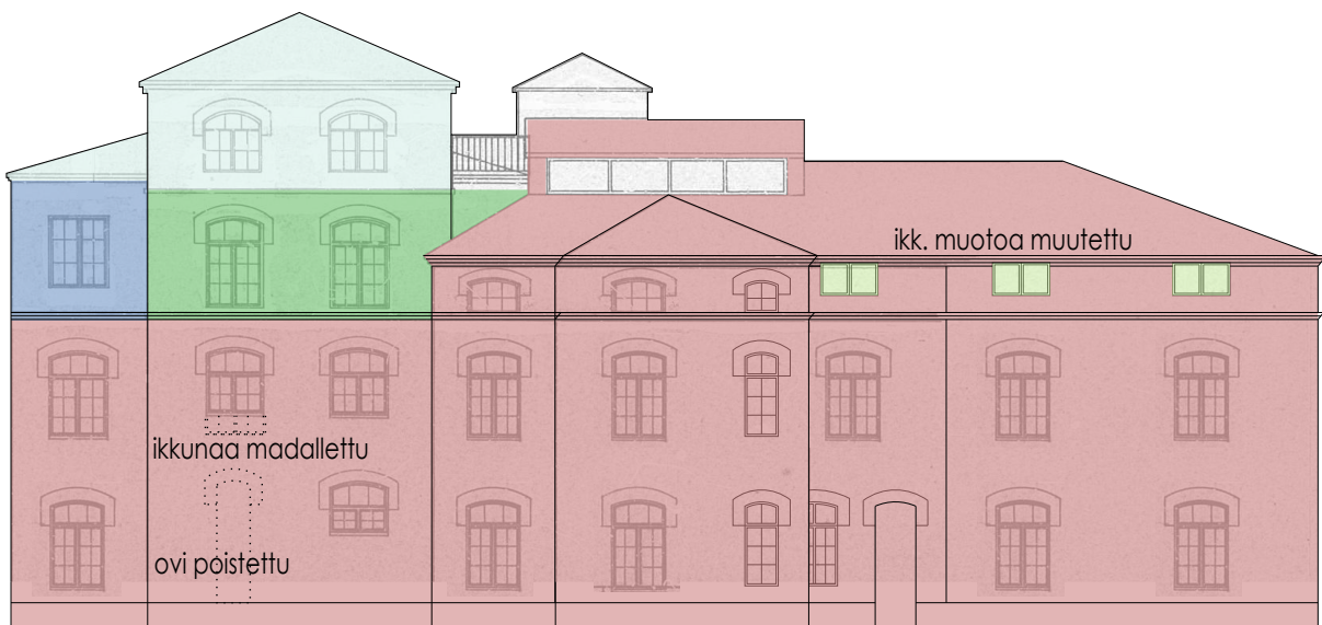
JULKISIVU POHJOISEEN
