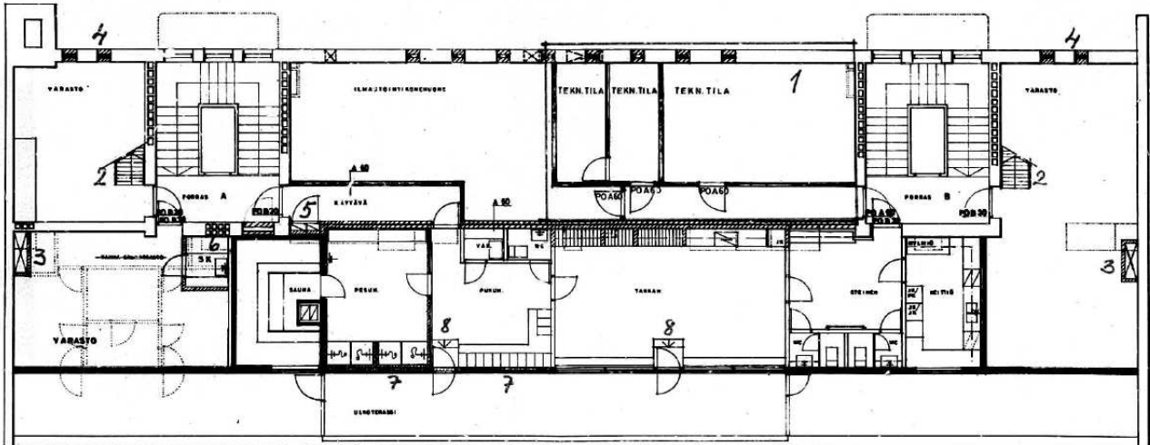
Pohjapiirros ullakko – Ullakolle lisätty teknisiä tiloja ja rakennettu uusi suurempi saunoosasto. (Edellinen sauna vuodelta 1968.) Rakennuslupapiirustus, Antti Tähtinen 1976/ 1980.
