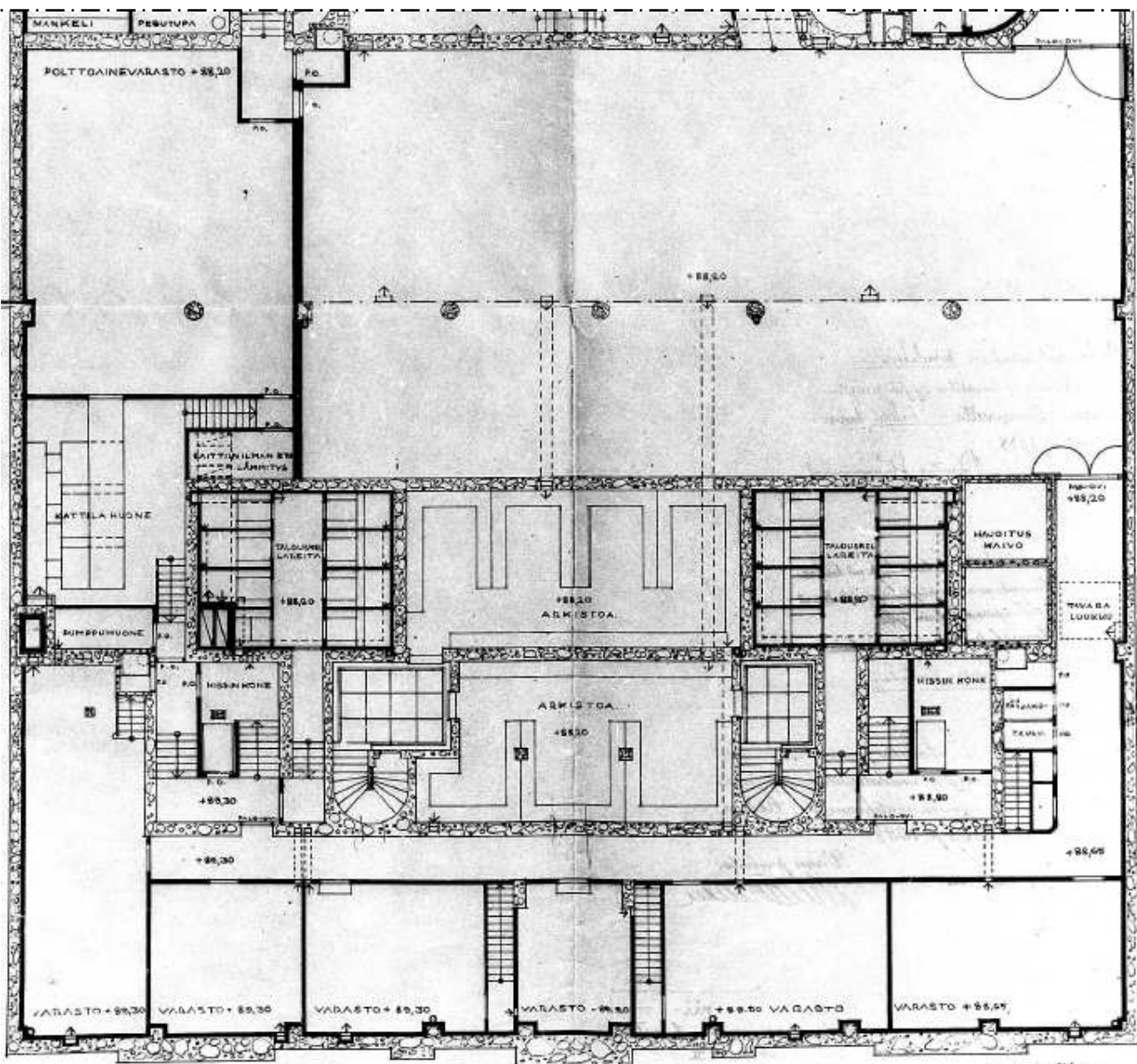
Yhdyspankintalon ullakon ja kellarin pohjapiirrokset. Rakennuslupapiirustus, Jaakko Tähtinen 1937.
