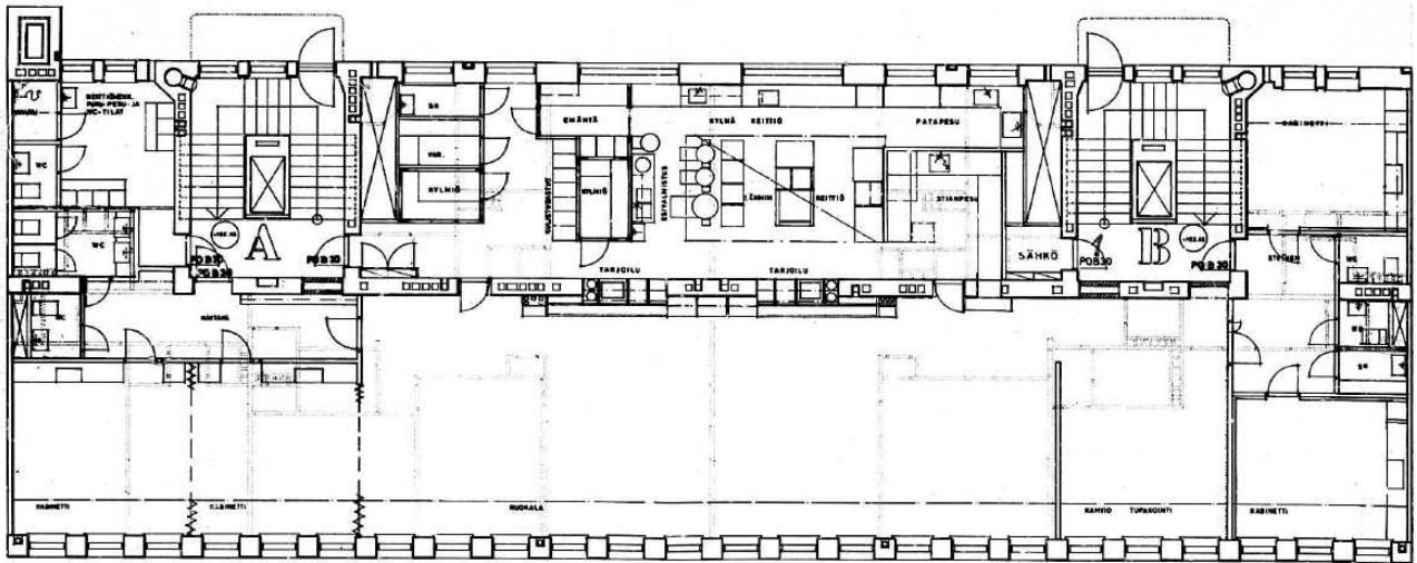
Pohjapiirros 4.krs – asuinkerros muutettu henkilökunnan ruokalaksi, keittiöksi ja kabineteiksi. Rakennuslupapiirustus, Antti Tähtinen 1976/ 1980
