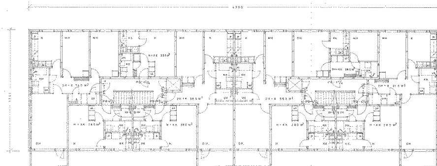
Kuva 18. Tontti 42. 1.-7. kerroksen pohjapiirros. Ei mittakaavassa. Kuva RaVa.
