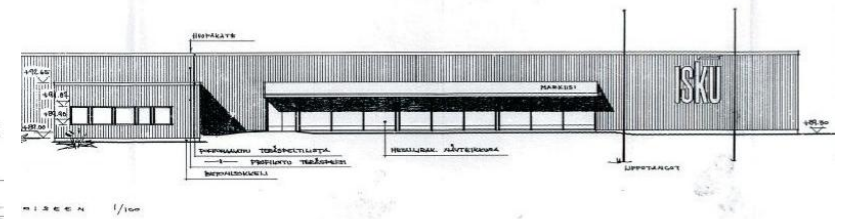
Eero Heleniuksen suunnittelema Kaiharin Kulma Oy:n julkisivu pohjoiseen 1970. Tampereen kaupungin rakennusvalvonnan piirustusarkisto.
