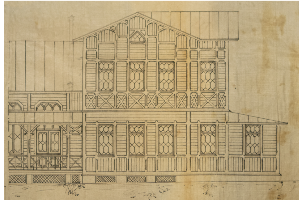
Julkisivu itään. Lambert Pettersonin huhtikuu 1900. TPA.
