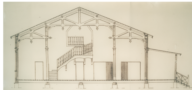
Leikkaus 15.4.1978. TPA.
