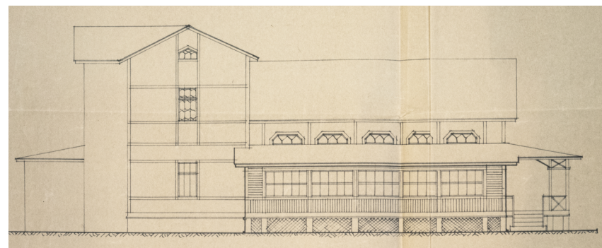
Länsijulkisivu syyskuussa 1932. TKA.
