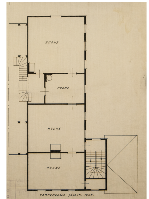
Ravintolan yläkerran pohjapiirros joulukuussa 1924. TPA.
