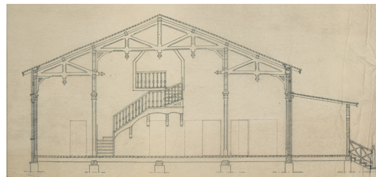
Leikkaus 11.6.1991. Teuvo Viitanen. TPA.
