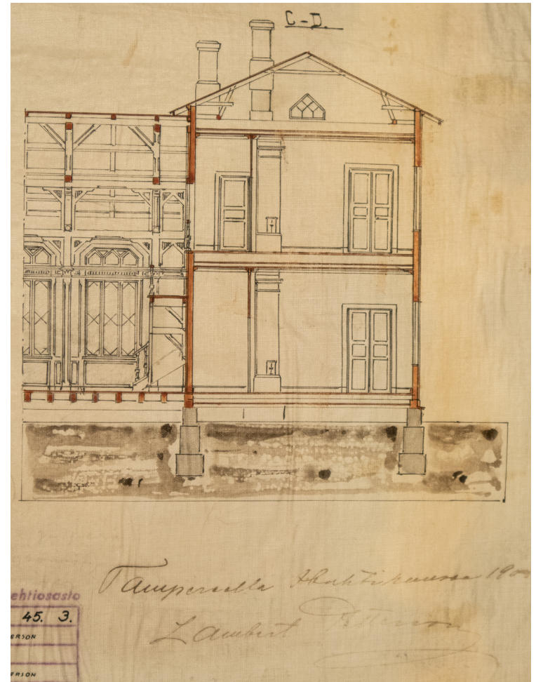
Lambert Petterssonin leikkauspiirustus ravintolasta. Huhtikuu 1900. TPA.
