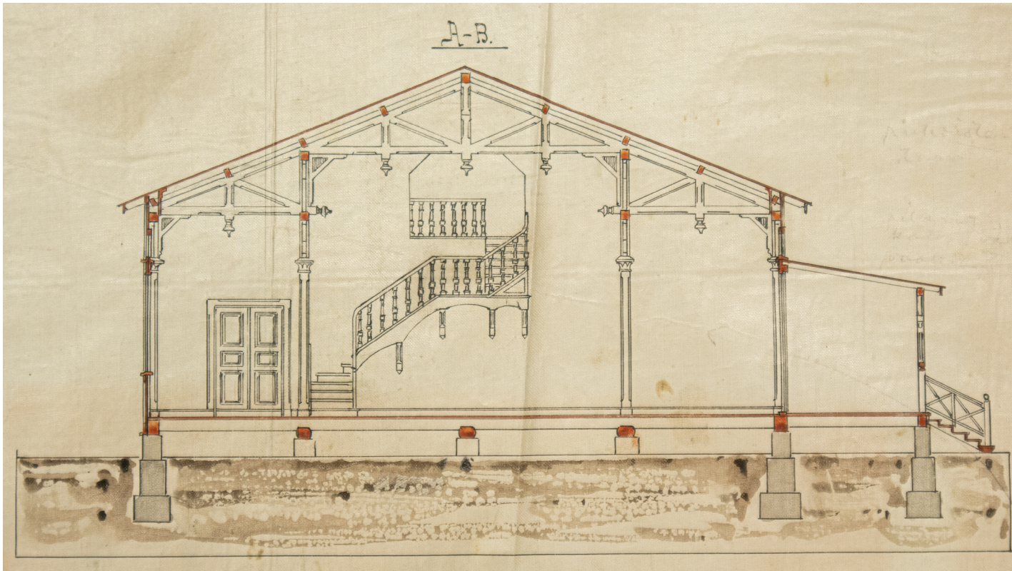
Leikkaus A-B. Lambert Petterson huhtikuu 1900. TPA.
