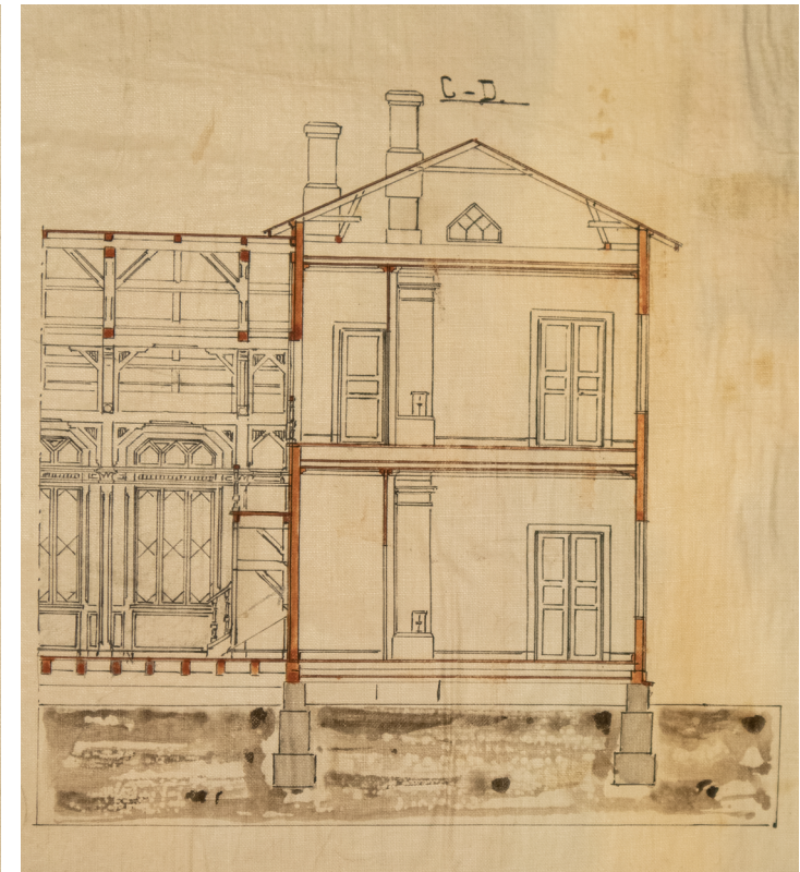
Leikkaus C-D. Lambert Petterson huhtikuu 1900. TPA.
