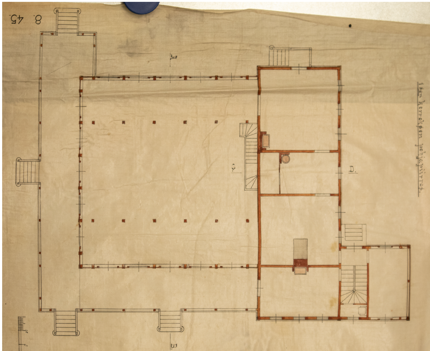
Pääkerroksen alkuperäinen pohjapiirros. Lambert Petterson huhtikuu 1900. TPA.
