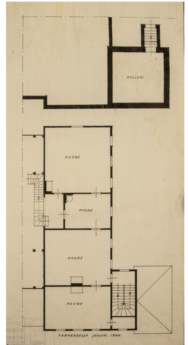
Vanhin säilynyt pohjapiirros ravintolan kellarista ja yläkerrasta. Tampereella joulukuussa 1924.TPA.
