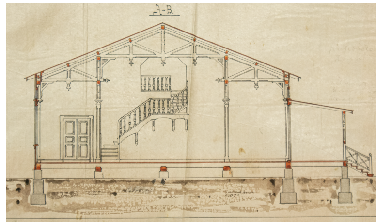
Leikkaus A-B, huhtikuu 1900. Lambert Petterson. TPA.
