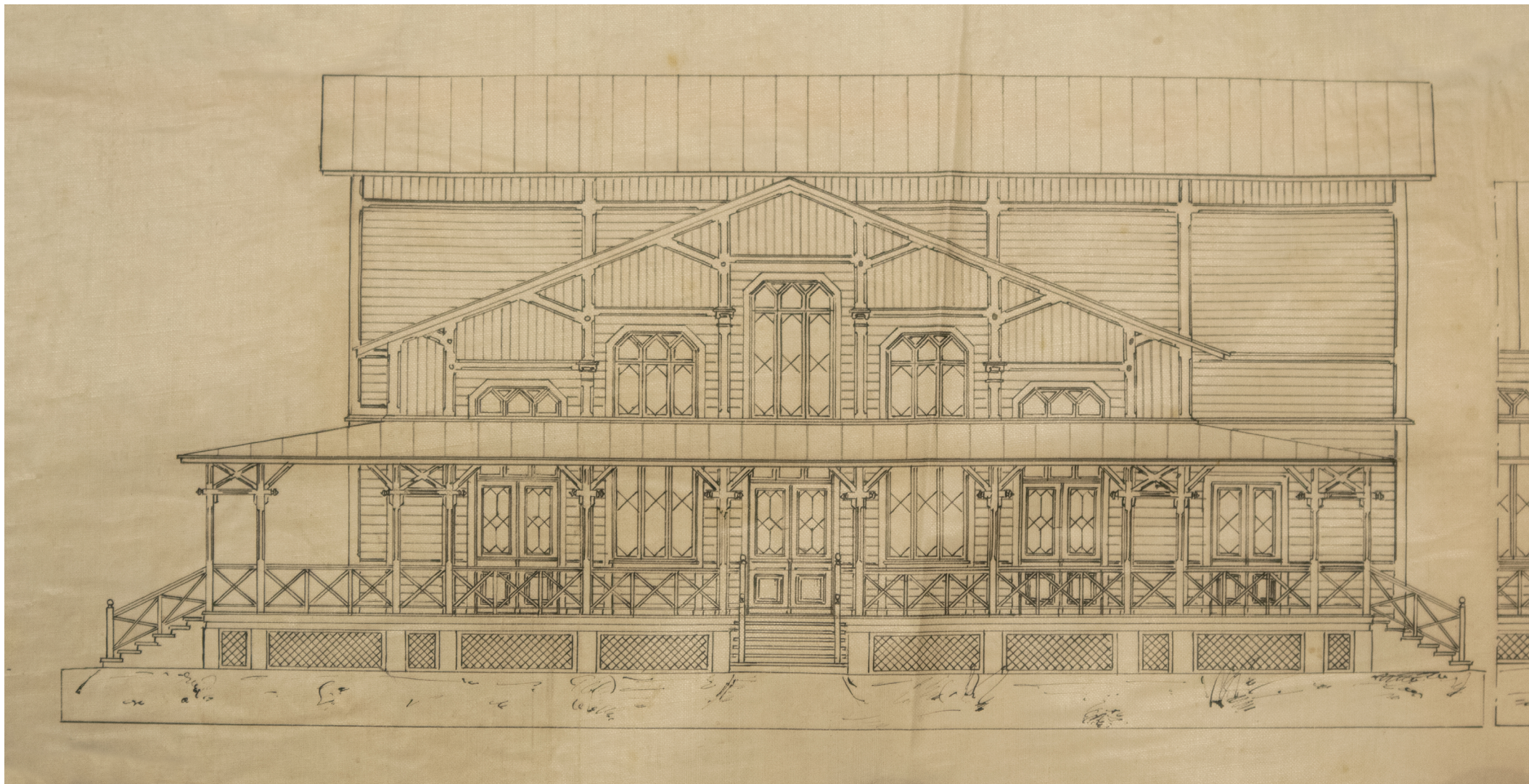
Julkisivu etelään. Lambert Petterson huhtikuu 1900. TPA.
