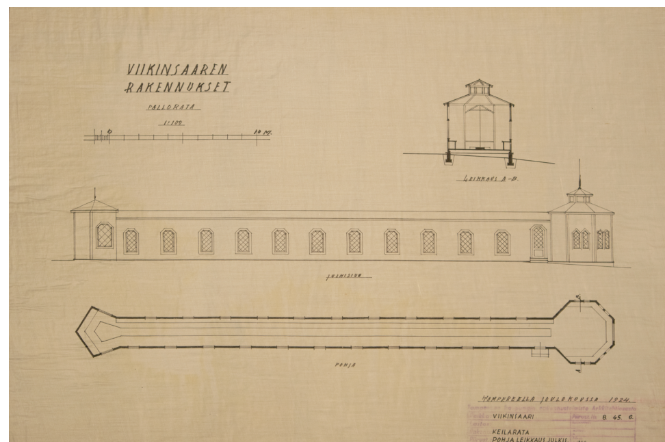
Joselinniemestä siirretty keilarata. Piirustus joulukuulta 1924. TPA.
