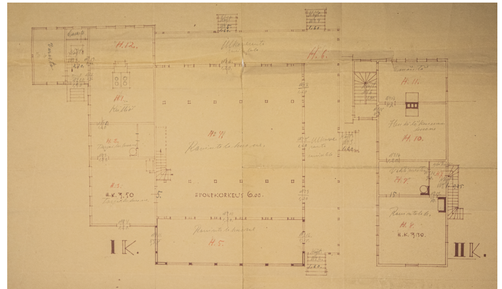
Ravintolan pohjapiirros. Tampereella syyskuussa 1932, TKA.
