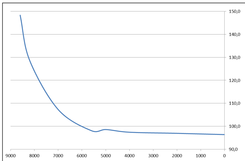
Näsijärven rannansiirtymiskäyrä Terälahdella (Jussila 2002, perustuen Tikkanen M & Seppä H, 2001: Postglacial history of Lake Näsijärvi, Finland, and the origin of the Tammerkoski Rapids. Fennia 179: 1 : 129-141 )
